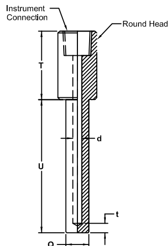
Straight Thermowell
