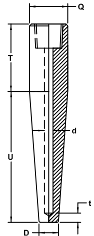
Taper Thermowell
