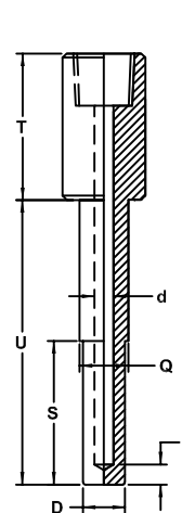
Step Thermowell
